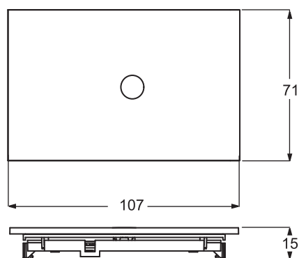
Inbouw-bewegingsmelder Busch-priOn® 6345-xxx-101
