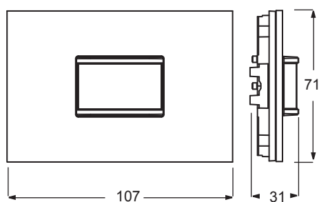
Inbouw-bewegingsmelder Busch-priOn® 6345-xxx-101
