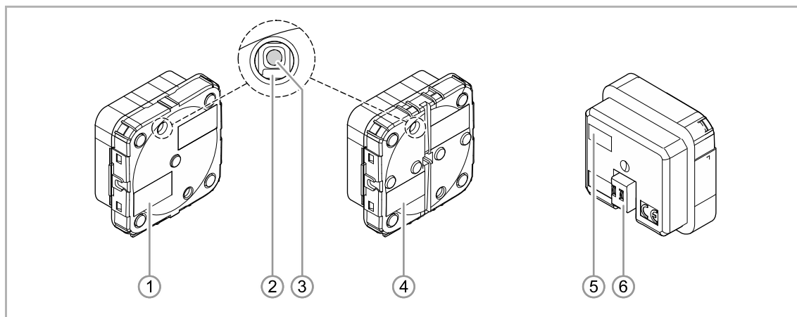
Afb. 2: Apparaatoverzicht
