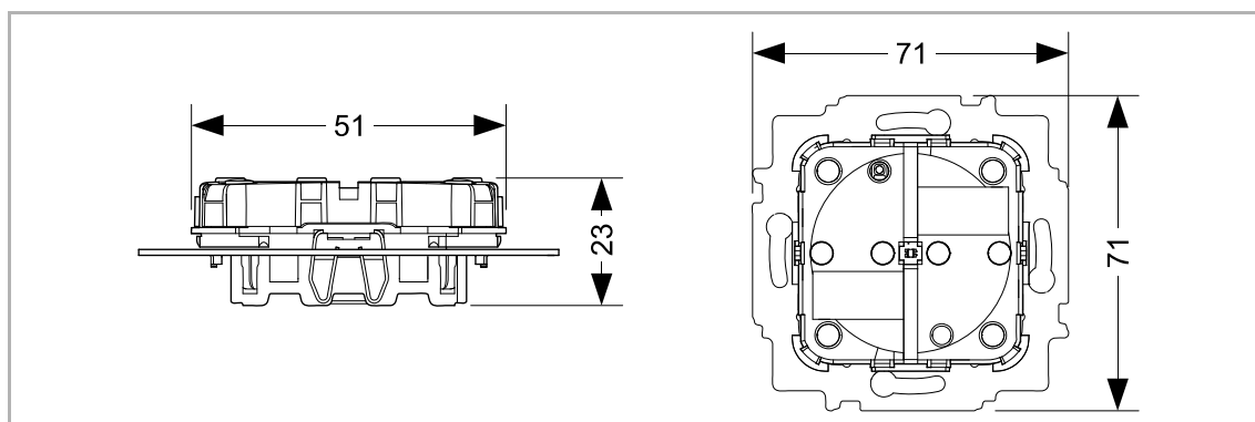
Afb. 3: Afmetingen (alle afmetingen in mm)
