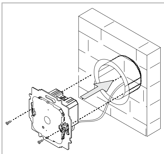
Fig. 11 : Monter le mécanisme encastré
