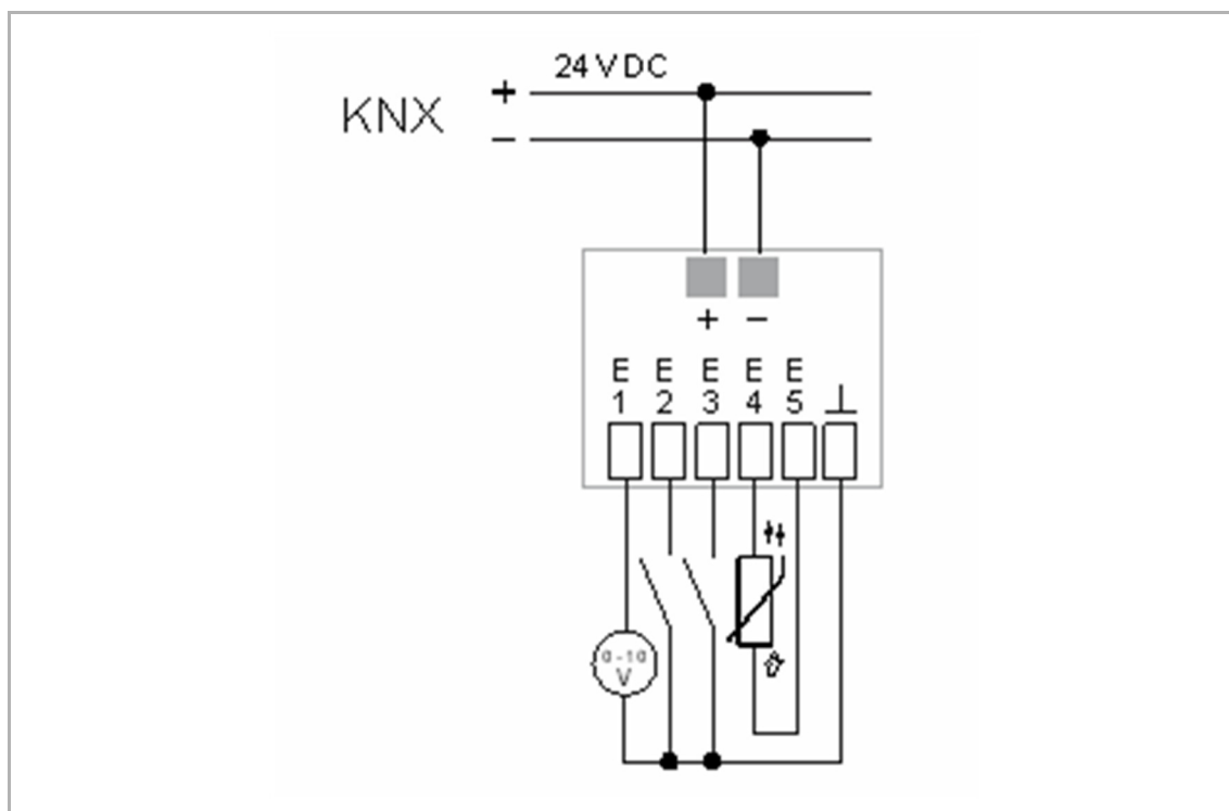
Fig. 14 : Raccordement électrique
