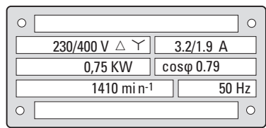
图片 19: 电机铭牌（标牌）示例
