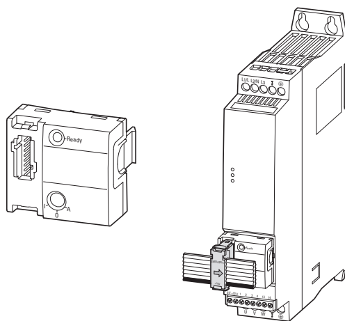
图片 59: SWD 连接组件 DX-NET-SWD3
