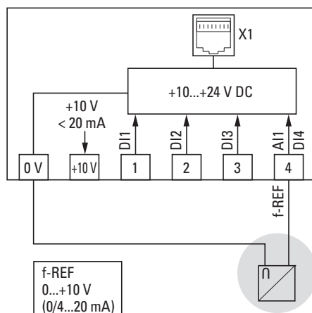
图片 40: 外部模拟额定值源的连接示例
