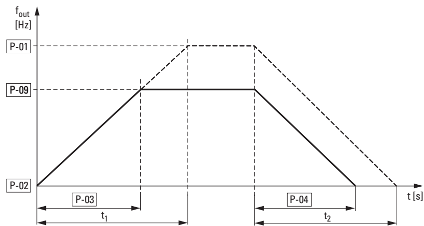
图片 62: 加速和减速时间
