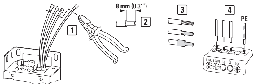
图片 84: 量产型连接导线的适配
