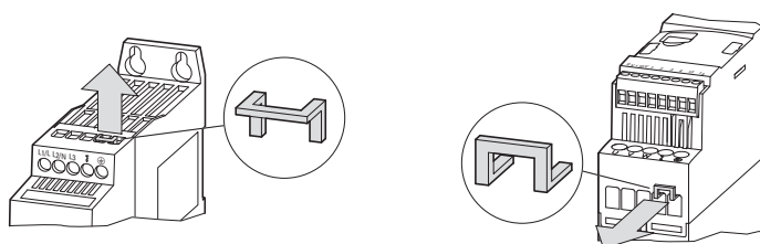
图片 34: 移除电网侧和电机侧的 EMC 电桥
