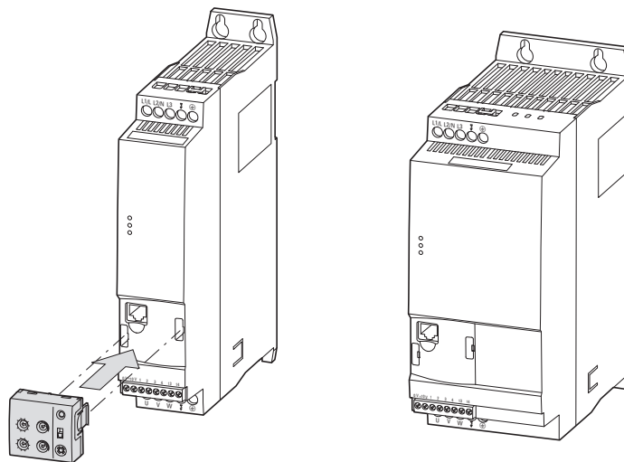
图片 1: DE1... 的壳体派生型（左侧：45 mm，右侧：90 mm）和可选配置模块 DXE-EXT-SET
