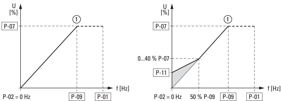
图片 66: U/f 特性曲线
