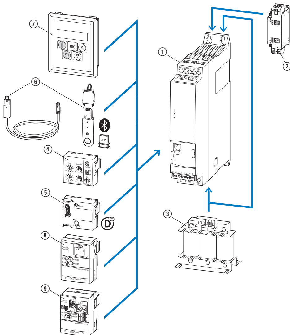
图片 2: 系统概览 (示例)
