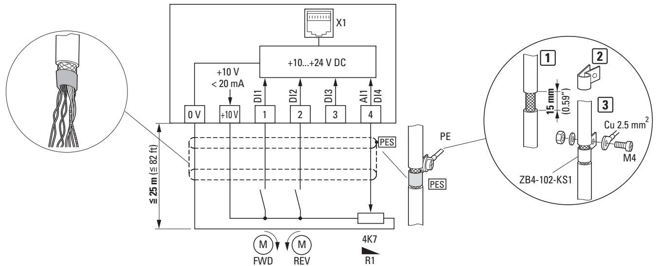
图片 39: 控制端子的连接示例
