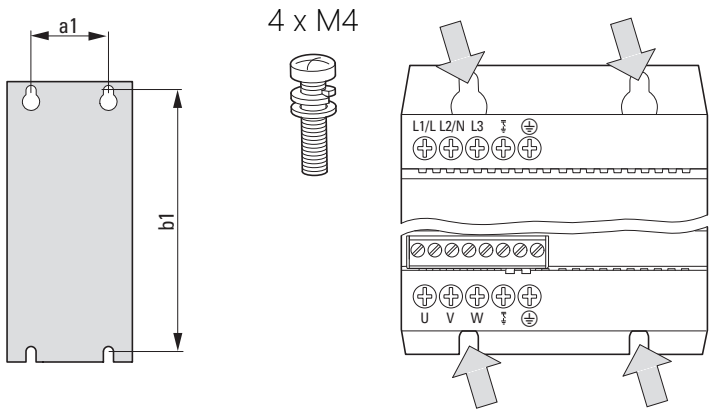
图片 25: 螺丝固定
