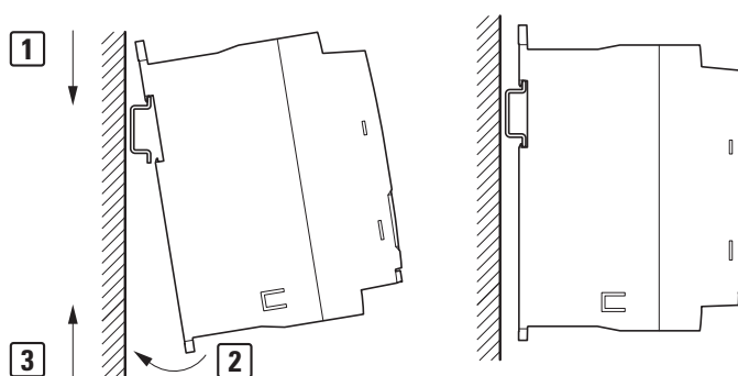
图片 27: 装配轨道固定
