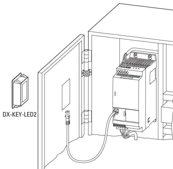
图片 73: 开关柜门中的装配
