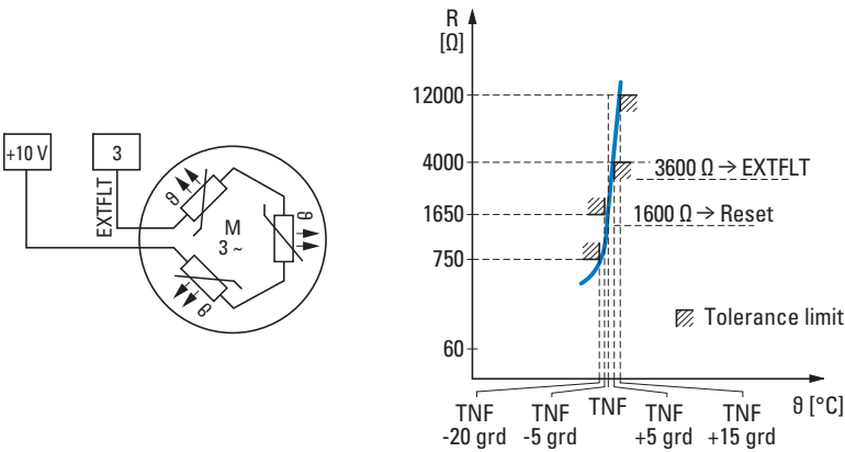
图片 65: 热传感器的连接示例和触发特性曲线
