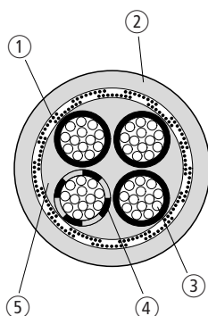
图片 37: 四线屏蔽型电机导线
