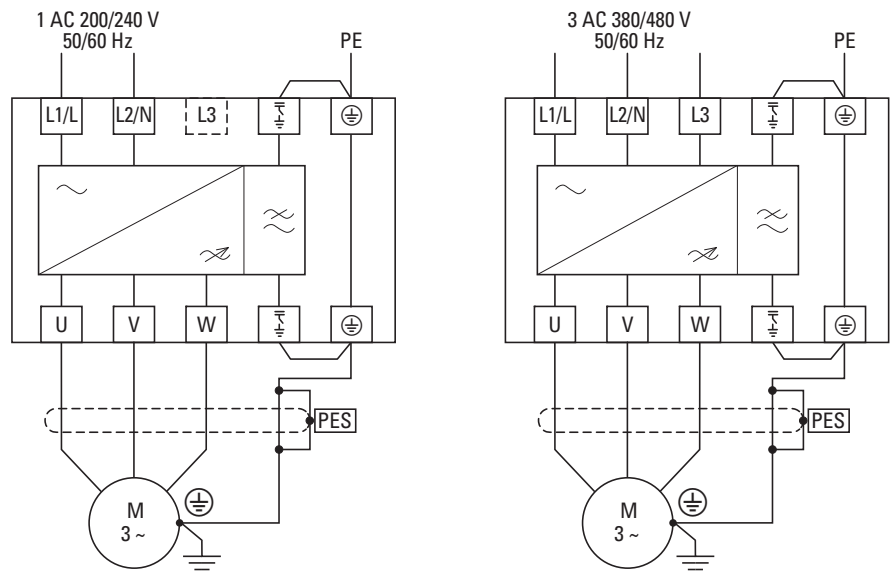
图片 29: 功率件内的连接（原理）
