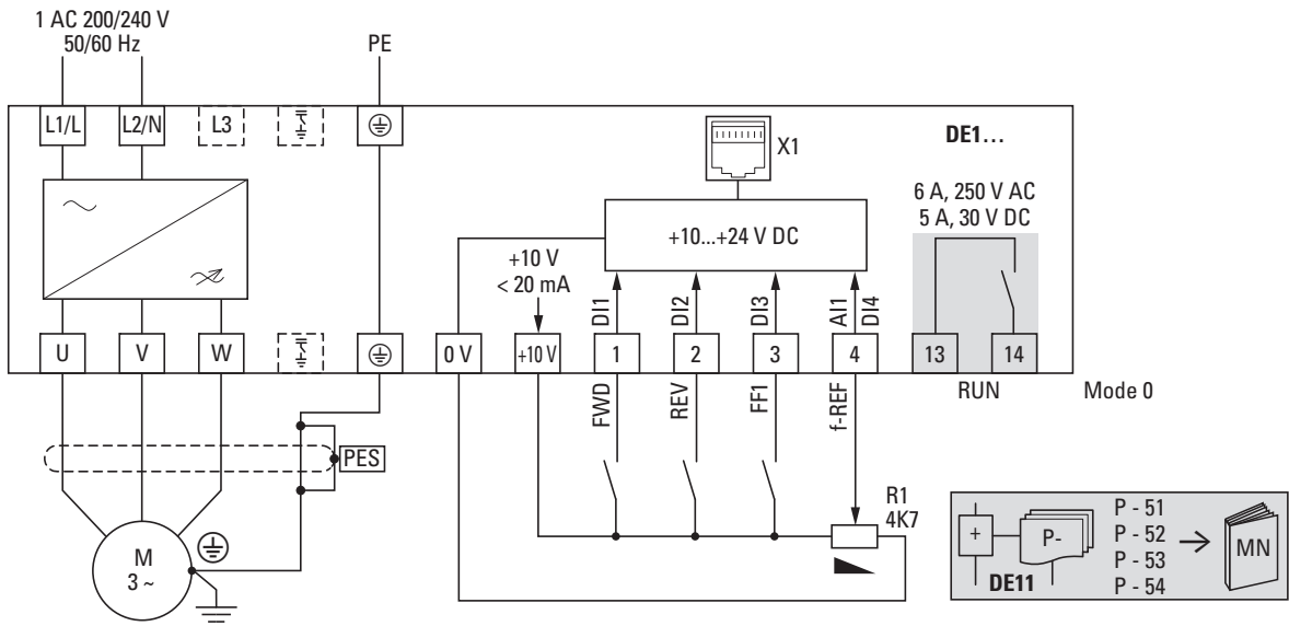
图片 47: 模块电路图 具有单相电网供电电压，无内部射频干扰滤波器的变速驱动器 DE1-12...NN-...
