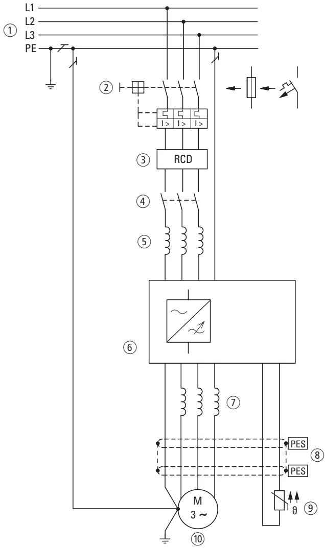
图片 14: 配备三相供电装置的驱动系统示例， 用于三相交流电机
