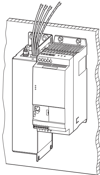
图片 83: 装配置 (例如: DX-EMC34-019... 和 DE1...-340... 采用规格 FS2)
