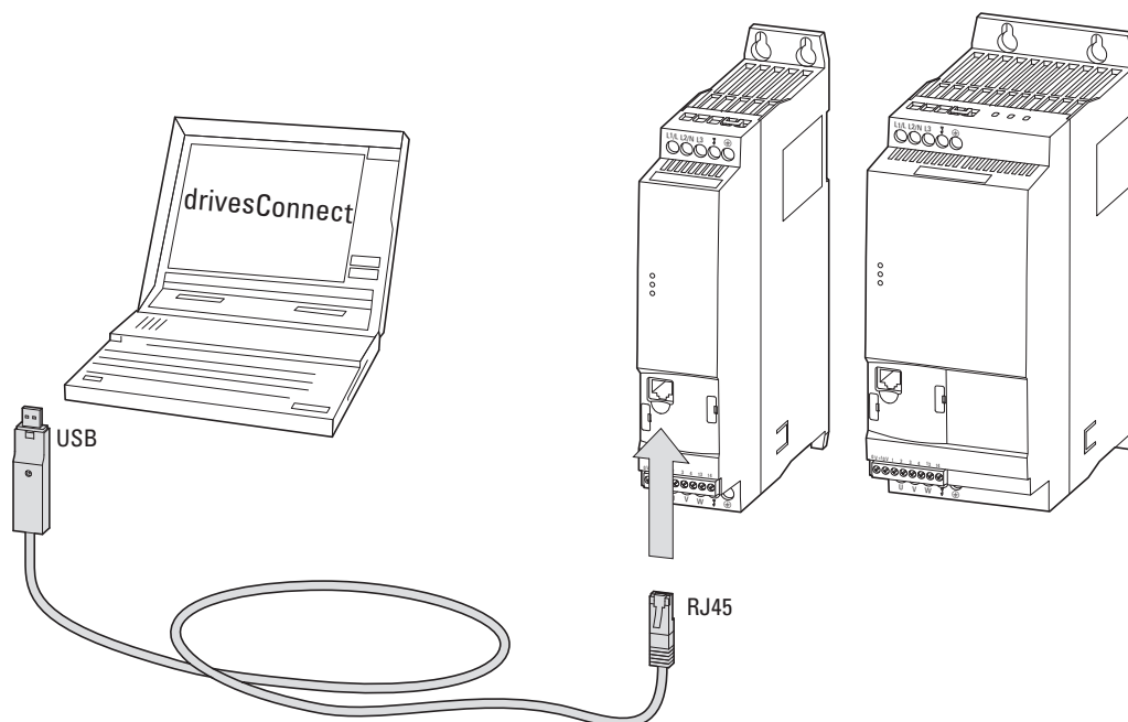
图片 79: DX-CBL-PC-3M0
