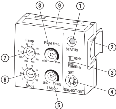
图片 51: DXE-EXT-SET 上各功能按键的名称
