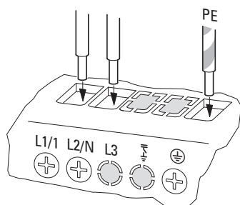
图片 30: 封闭的连接端子（例如：DE1-12...NN-...）
