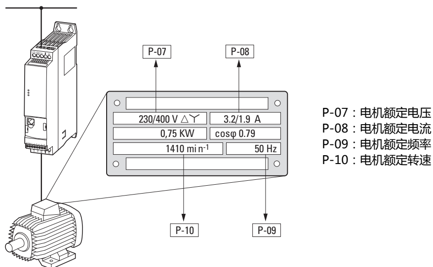
图片 13: 选择标准
