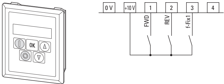
图片 70: 选配的操作单元 DXE-KEY-LED2 和控制端子 P-15 = 0（出厂设置，模式 0）
