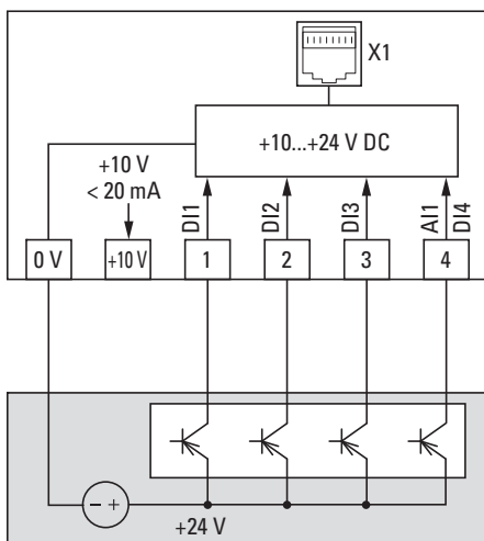
图片 72: 外部控制示例
