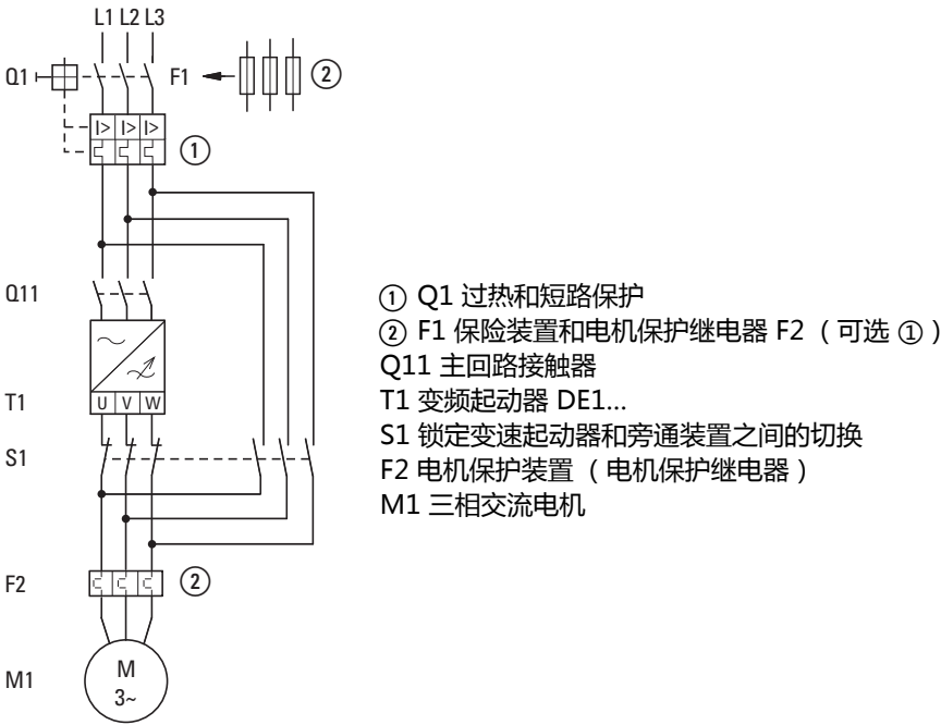
图片 16: 旁通电机控制装置（示例）
