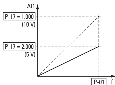
图片 71: 缩放的额定值输入端
