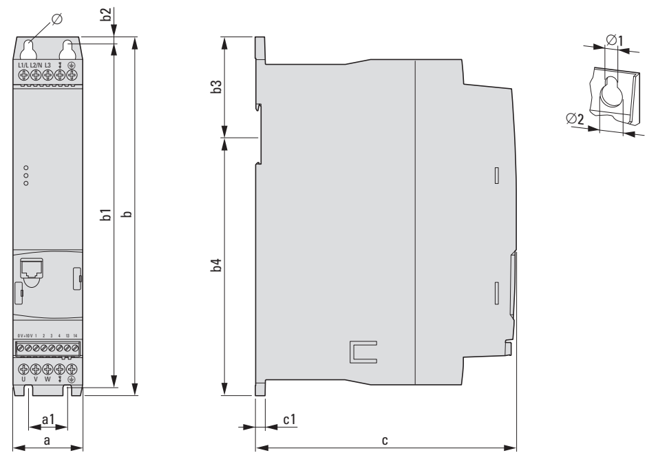
图片 71: 尺寸
