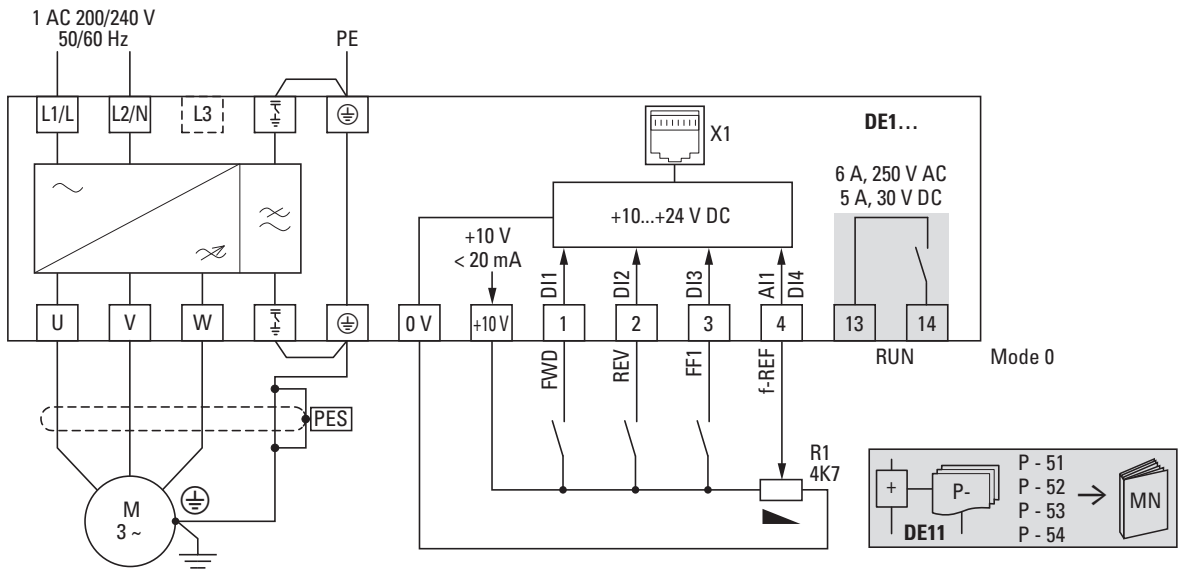
图片 46: 模块电路图 具有单相电网供电电压和内部射频干扰滤波器的变速驱动器 DE1-12...FN-...
