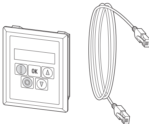
图片 72: DX-KEY-LED2 配备 RJ45 电缆 (3 m)
