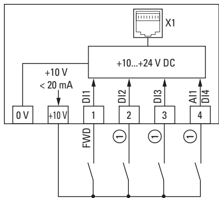
图片 41: 四个数字输入端的连接示例
