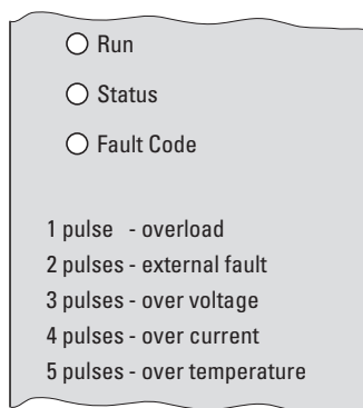
图片 45: 带有故障代码（壳体压印）的 LED 指示灯
