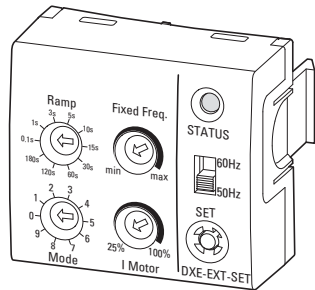
图片 50: 配置模块 DXE-EXT-SET
