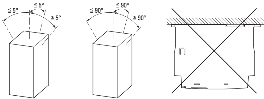
图片 22: 安装位置 ( 左侧 : 设备 DE1...-121D4, DE1...-122D3... 和 DE1...-122D7...)
