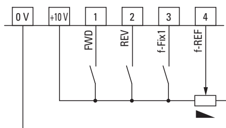
图片 68: 控制端子的出厂设置
