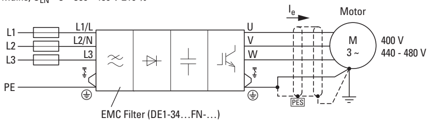
图片 11: DE1...-34...FN-N20N (带有射频干扰滤波器)
