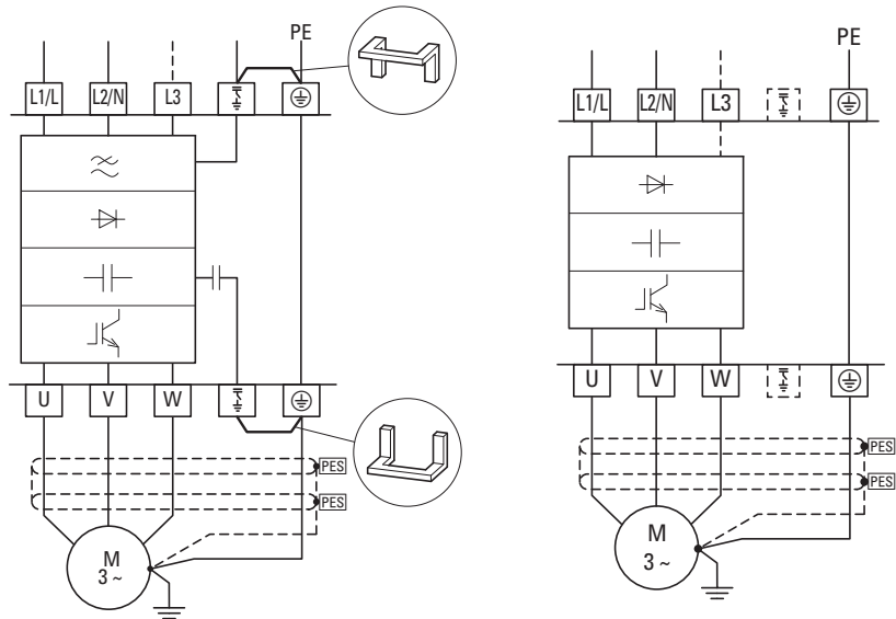
图片 33: DE1...-...FN-...（带有滤波器） DE1...-...NN-...（不带滤波器）
