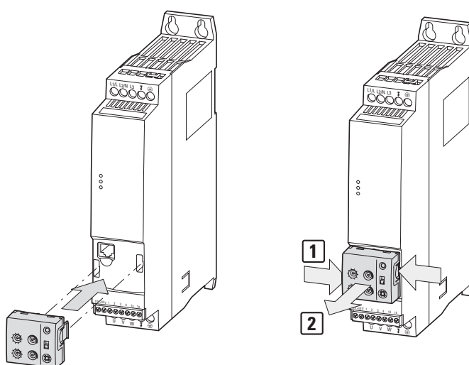
图片 52: 装配和拆卸
