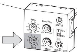
图片 69: 配置模块 DXE-EXT-SET
