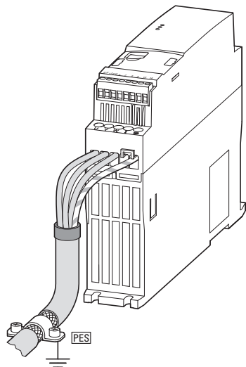
图片 35: 电机侧连接
