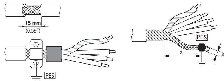
图片 36: 电机电路中屏蔽型连接导线
