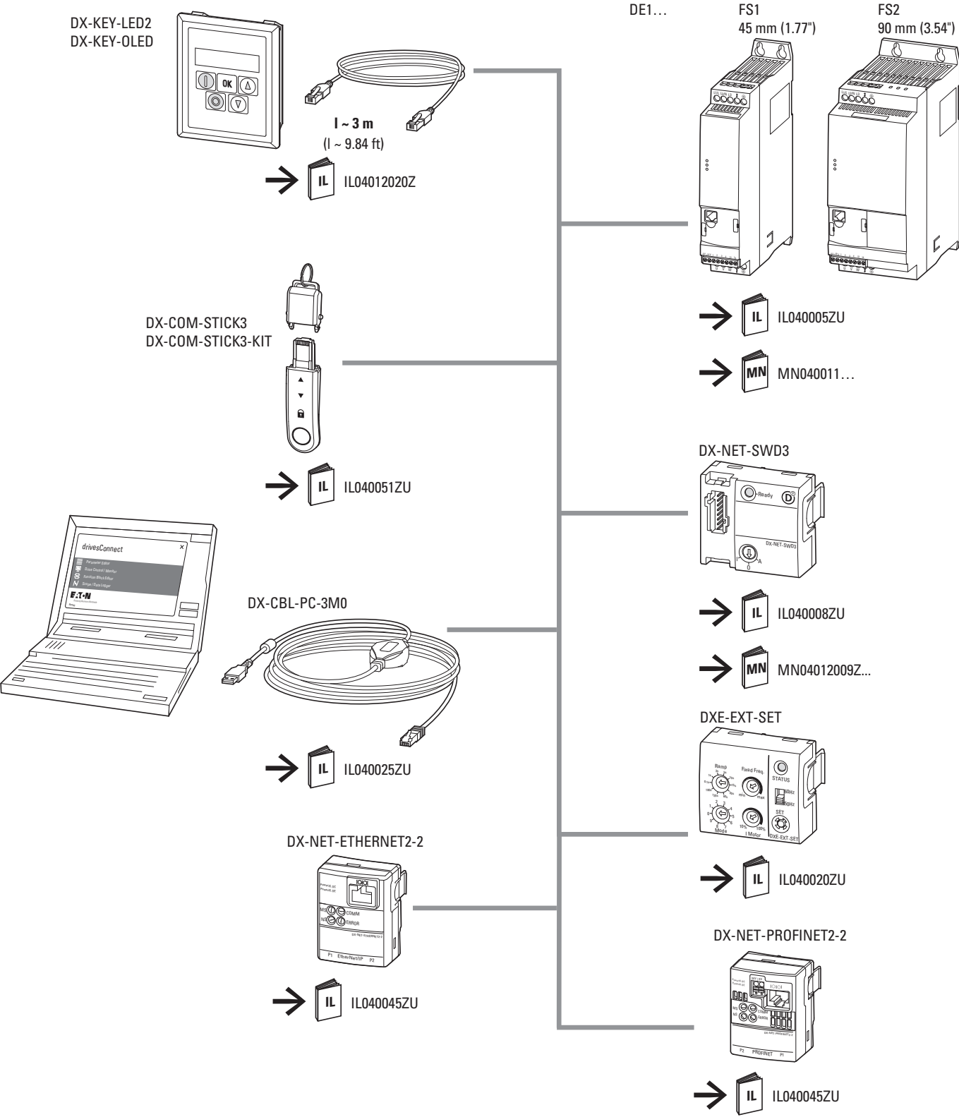
图片 44: 变频起动器 DE1 的 RJ45 接口的系统概览
