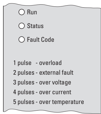
图片 86: 带有故障信息的 LED 指示灯
