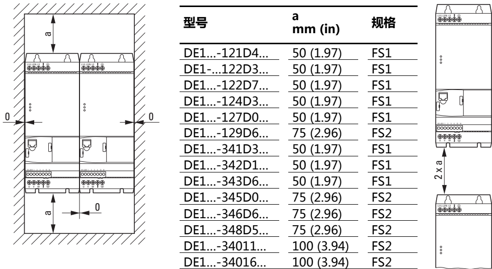
图片 23: 用于空气冷却的自由空间
