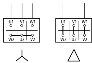
图片 20: 接线方式： 星形电路（左），三角电路（右）
