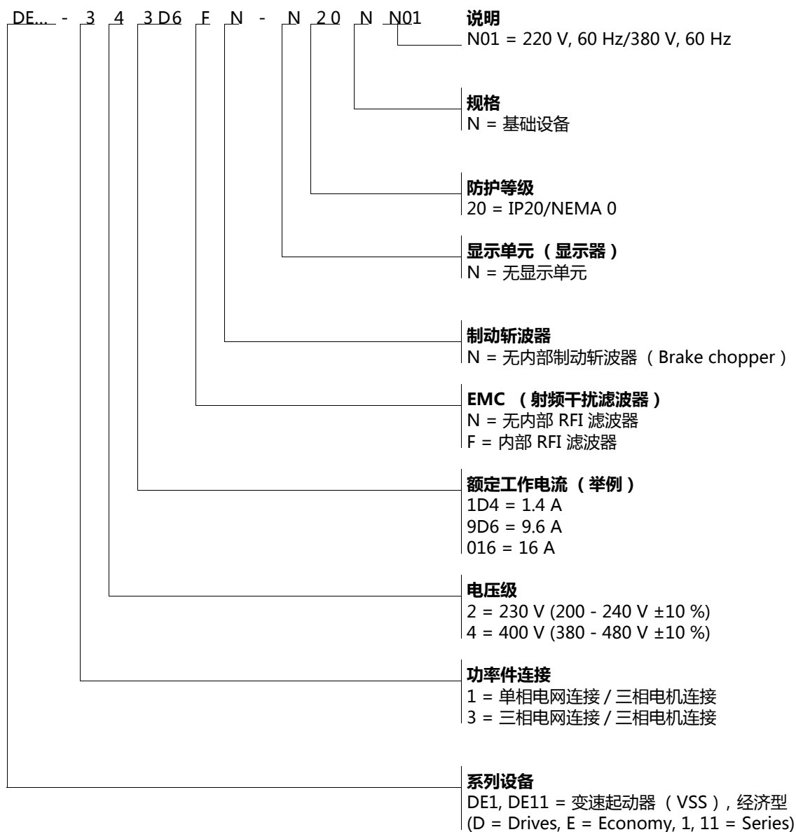
图片 7: 型号代码
