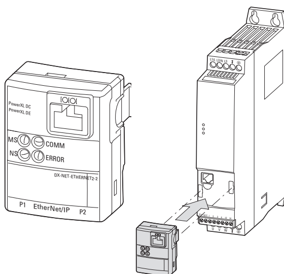
图片 60: EtherNet/IP 连接组件 DX-NET-ETHERNET2-2
