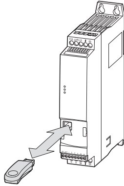
图片 75: DE1... 和 DX-COM-STICK3
