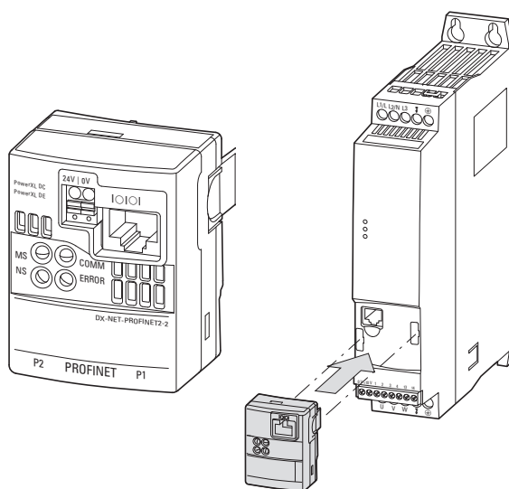
图片 61: PROFINET 连接组件 DX-NET-PROFINET2-2
