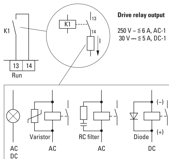
图片 42: 带有保护线路的连接示例
