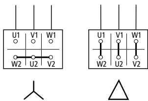
图片 64: 接线方式（三角形，星形）
