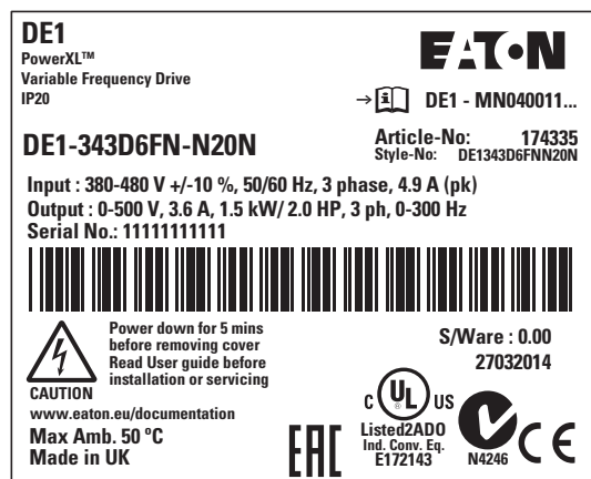
图片 5: 铭牌 A（安装于侧面）
