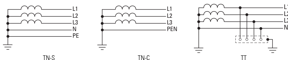
图片 15: 中点接地的交流电网
