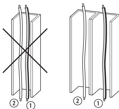
图片 18: 独立的导线布线
