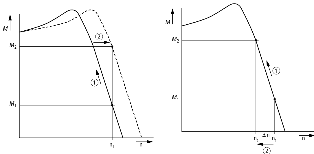
图片 67: 带有和不带滑差补偿的转速特性。
