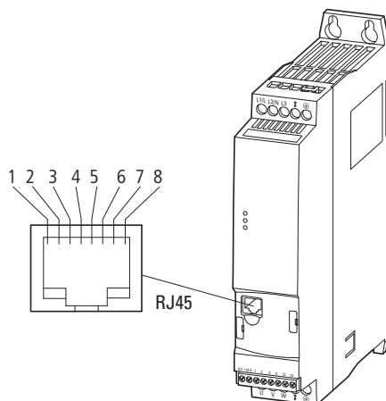
图片 54: RJ45 接口
