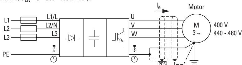
图片 12: DE1...-34...NN-N20N (不带射频干扰滤波器)
