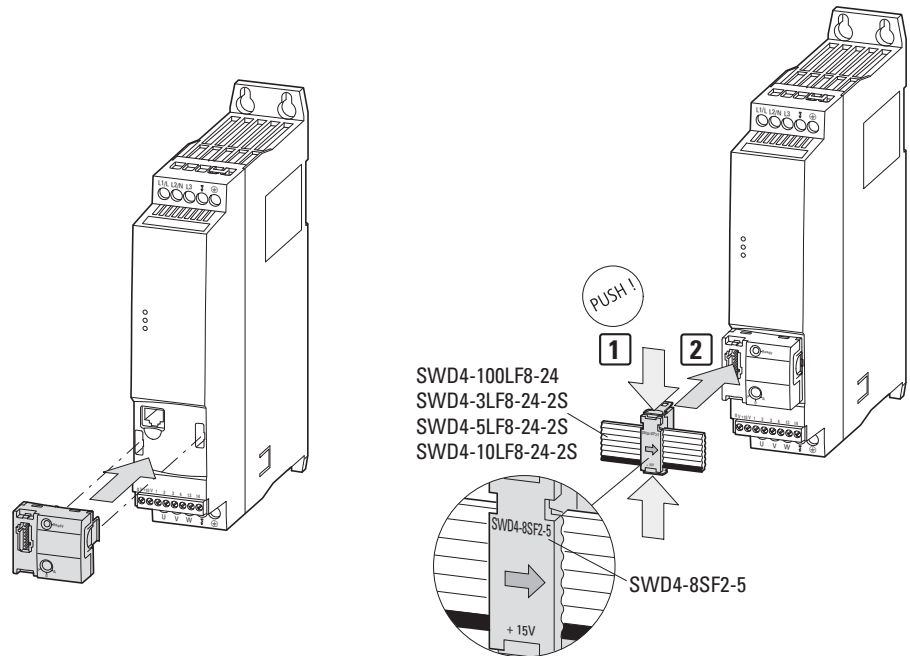
图片 78: SmartWire-DT 连接
