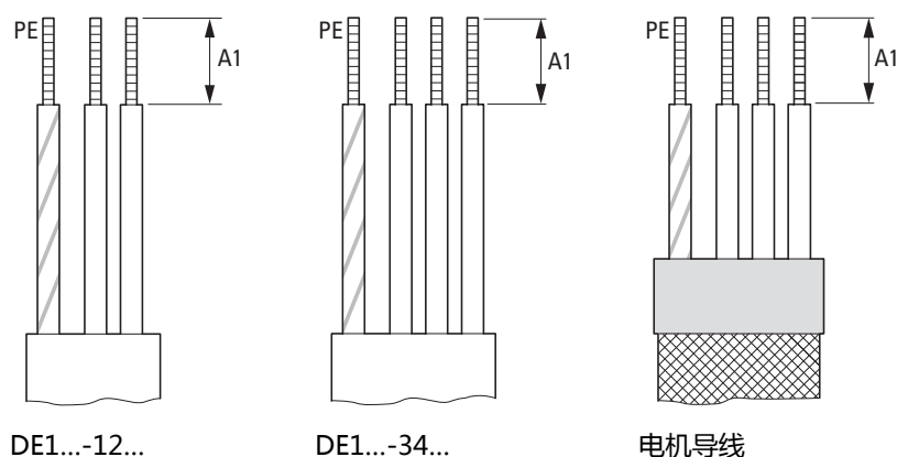
图片 31: 功率件内的剥线长度
