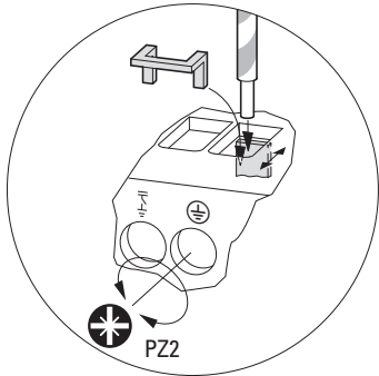
图片 32: PE 导线插入 EMC 电桥后部 (由后至前夹紧)
