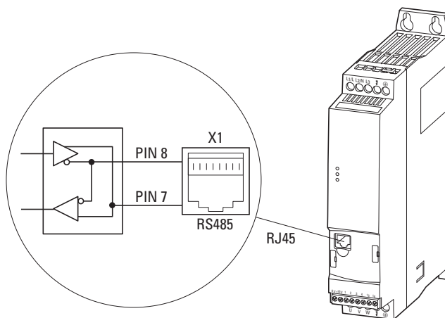
图片 43: RJ45 接口
