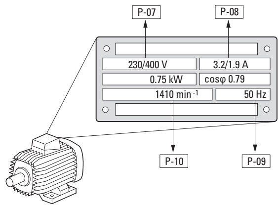
图片 63: 标牌上的电机参数
