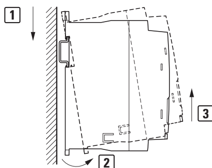
图片 28: 装配轨道的拆卸
