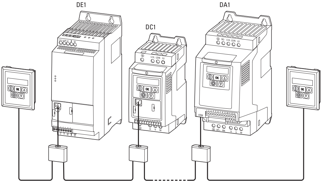
图片 74: 示例：带有两个操作单元的 PowerXL 网络（OP 总线）
