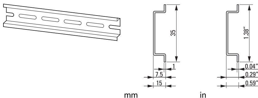
图片 26: 符合 IEC/EN 60715 标准的装配轨道
