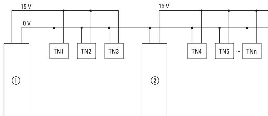
Abbildung 37: Schematischer Aufbau eines SWD-Strangs mit PowerFeed-Modul EU5C-SWD-PF2
