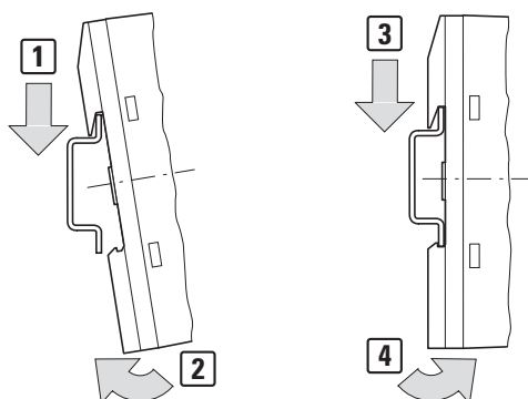
Abbildung 8: Montage auf Hutschiene
