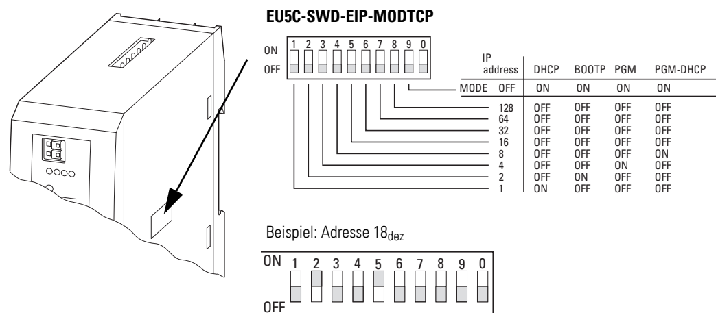
Abbildung 5: Feldbusadresse am Gateway EU5C-SWD-EIP-MODTCP einstellen
