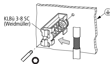
Abbildung 15: Abschirmung des Feldbusses durch Auflegen des Schirms
