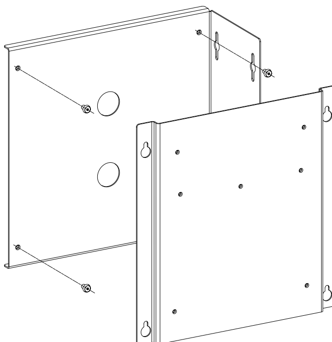
6169013 KV-HOUDER (OPTIONAL)
