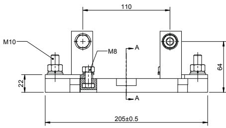
Dimensions (mm) - 170H3005
