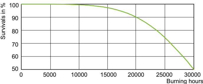
Life Expectancy Diagram - MASTER SON PIA Plus 70W E27
