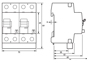
Maßzeichnung Gruppenansicht
