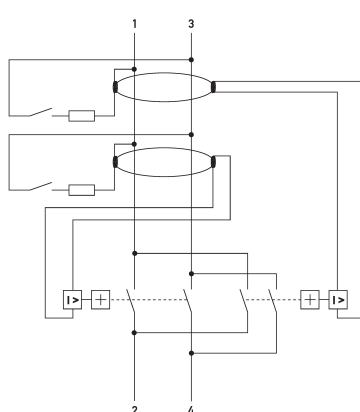
Anschlusschema
