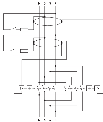
Anschlussschema
