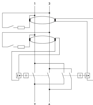
Anschlussschema
