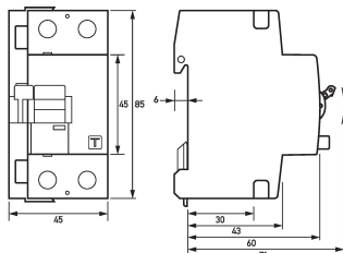
Maßzeichnung Gruppenansicht
