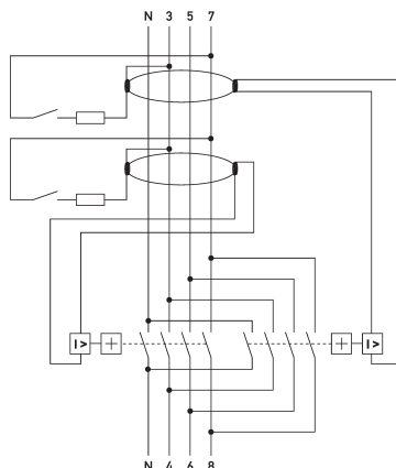
Anschlussschema
