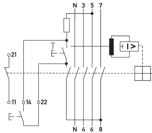
Anschlusschema
