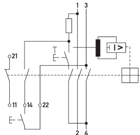
Anschlussschema
