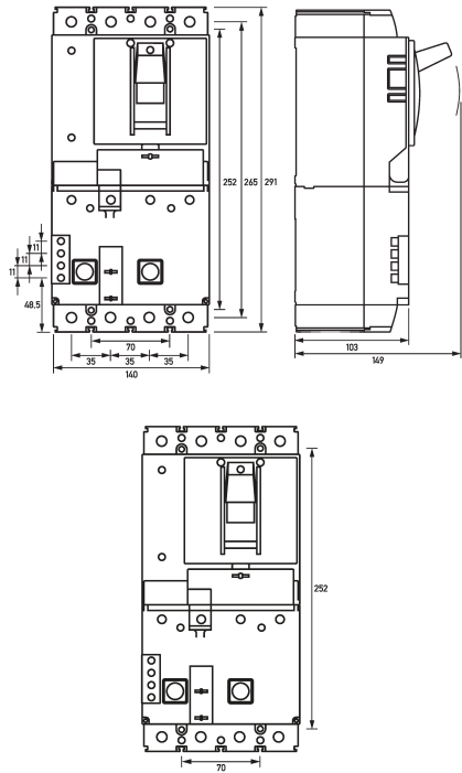
Maßzeichnung Gruppenansicht
