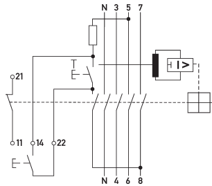
Anschlussschema
