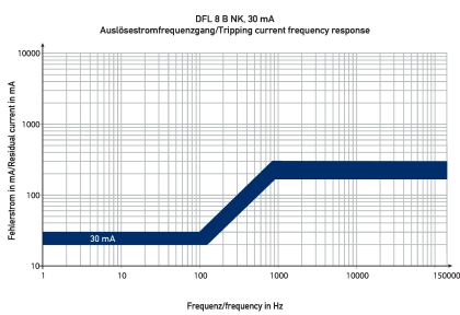
Kennlinie B NK 30 mA
