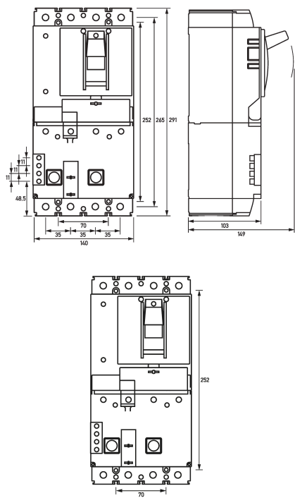
Maßzeichnung Gruppenansicht
