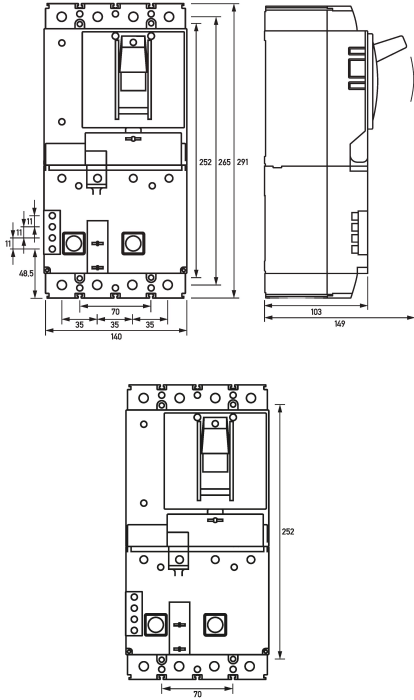
Maßzeichnung Gruppenansicht
