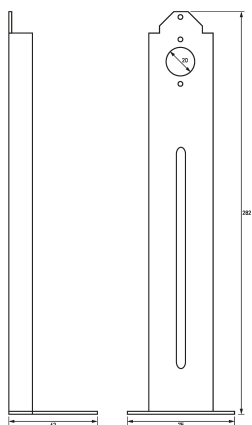
Maßzeichnung Gruppenansicht
