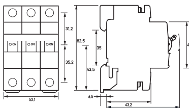
Maßzeichnung Gruppenansicht
