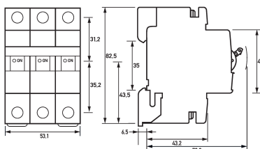
Maßzeichnung Gruppenansicht
