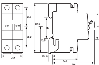
Maßzeichnung Gruppenansicht
