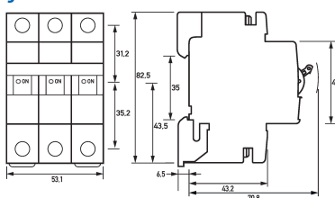
Maßzeichnung Gruppenansicht
