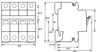
Maßzeichnung Gruppenansicht
