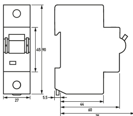
Maßzeichnung Gruppenansicht
