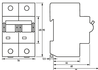
Maßzeichnung Gruppenansicht
