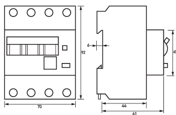
Maßzeichnung Gruppenansicht
