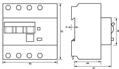
Maßzeichnung Gruppenansicht
