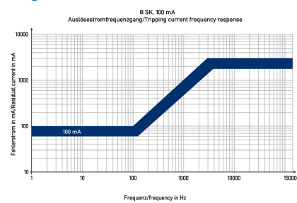
Kennlinie B SK 100 mA
