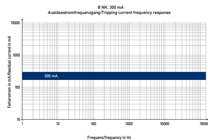
Kennlinie B NK 300 mA
