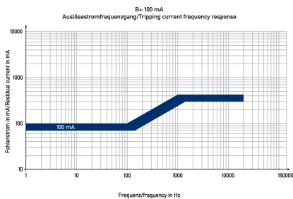
Kennlinie B+ 100 mA
