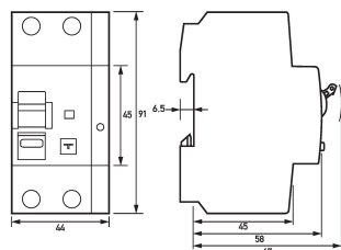
Maßzeichnung Gruppenansicht
