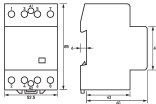
Maßzeichnung Gruppenansicht
