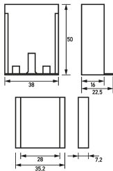
Maßzeichnung Gruppenansicht
