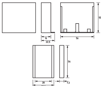
Maßzeichnung Gruppenansicht
