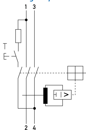
Anschlusschema
