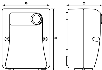
Maßzeichnung Gruppenansicht
