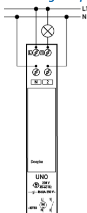
Schaltungsbeispiel
