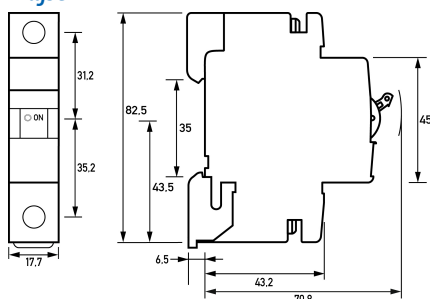
Maßzeichnung Gruppenansicht
