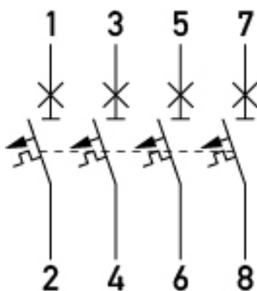
Anschlusschema
