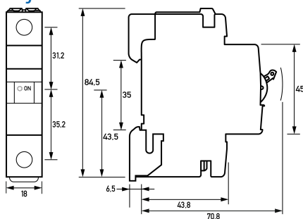
Maßzeichnung Gruppenansicht
