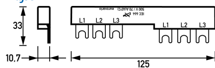
Maßzeichnung Gruppenansicht
