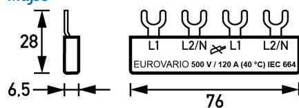
Maßzeichnung Gruppenansicht
