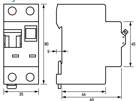
Maßzeichnung Gruppenansicht
