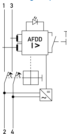
Anschlusschema
