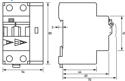
Maßzeichnung Gruppenansicht
