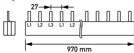
Maßzeichnung Gruppenansicht
