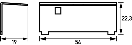
Maßzeichnung Gruppenansicht
