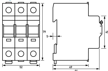
Maßzeichnung Gruppenansicht
