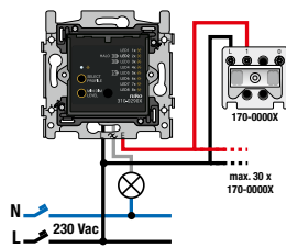
Mehrere Bedienungspunkte
